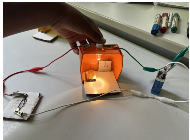
Ein kleines Zimmer für den Gummibär mit Schalter und stromsparender LED-Lampe
