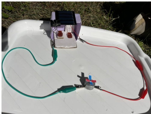
Gut zu wissen, wie ein Ventilator auch mit Solarenergie betrieben werden kann!
